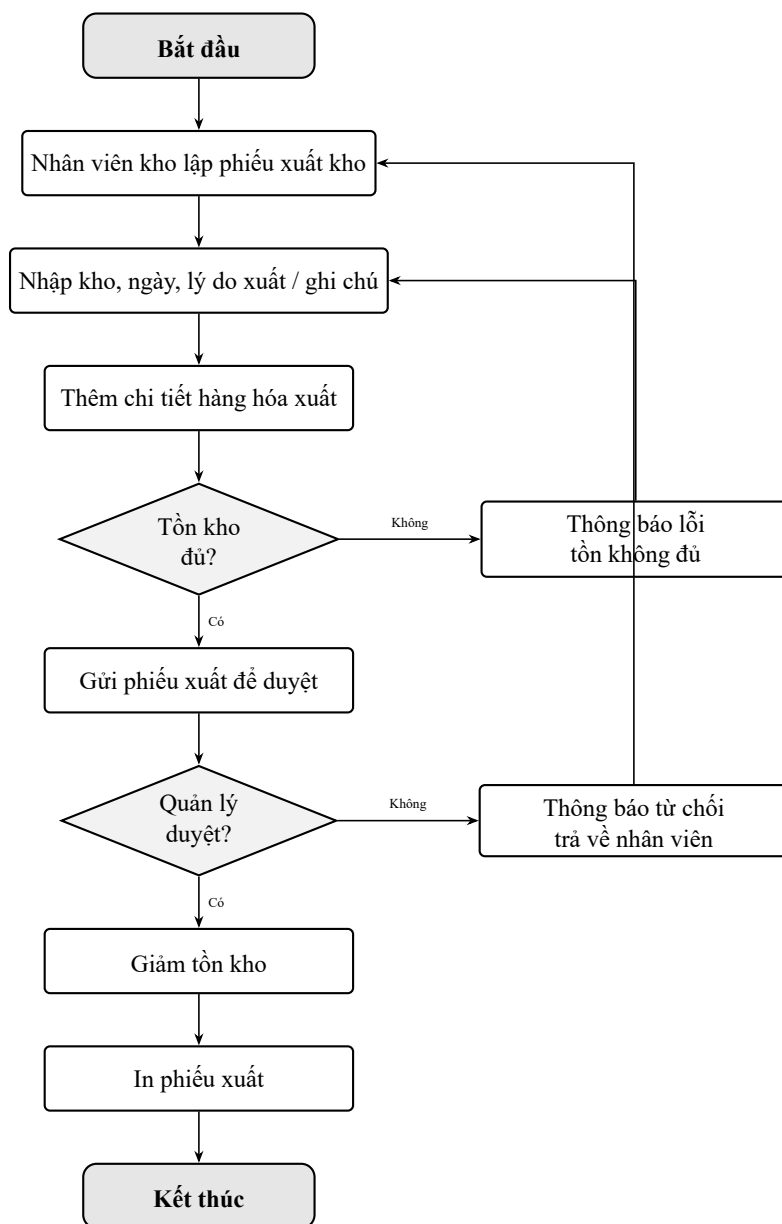
Hình 1: Activity – UC28 Lập phiếu xuất kho
